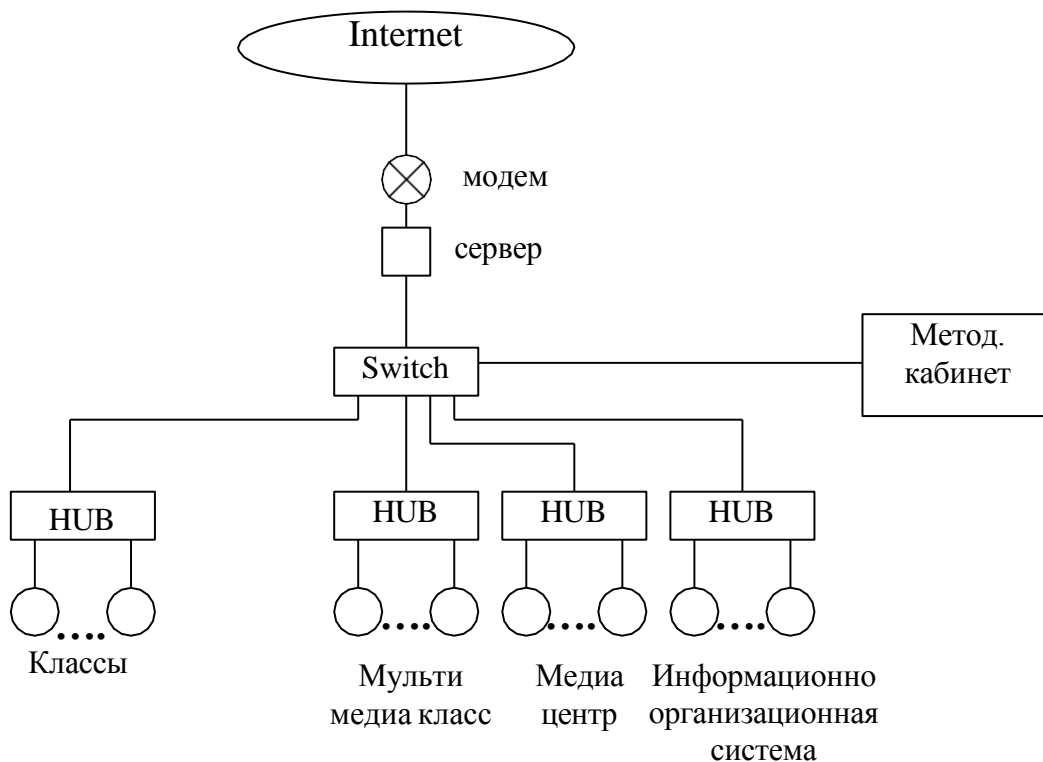
Схема предполагаемой сети
