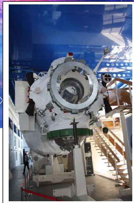
Комплекс макетов модулей орбитальной станции «Мир»
